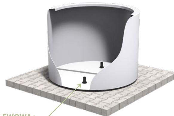
RURA PRZELEWOWA
